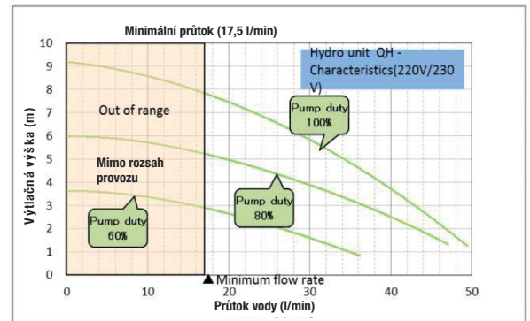
Charakteristika čerpadla HWS-1404XWH (11,14,16 kW)
