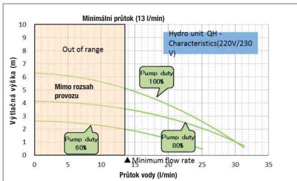
Charakteristika čerpadla HWS-804XWH (8kW)
